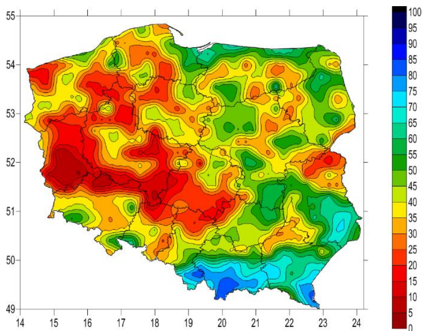
Wskaźnik wilgotności gleby w II połowie sierpnia (warstwa 7-28 cm)
